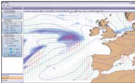
UGrib-Software
